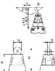
LXP1-120/G, J, H, K
